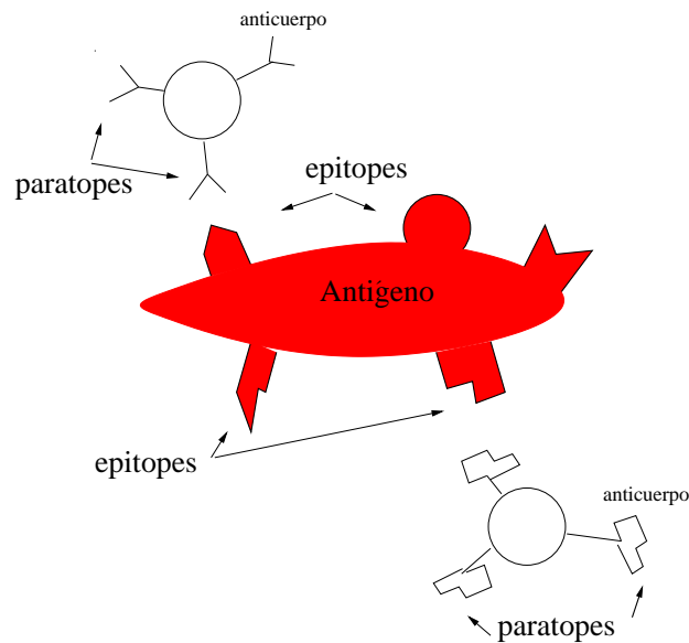
Figura 2.8: Relación paratope-epitope
